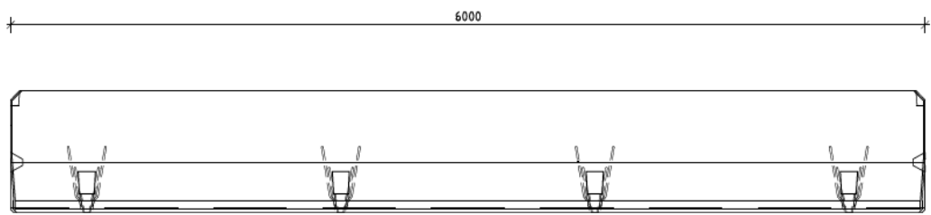
VOORAANZICHT SCHAAL 1:25
