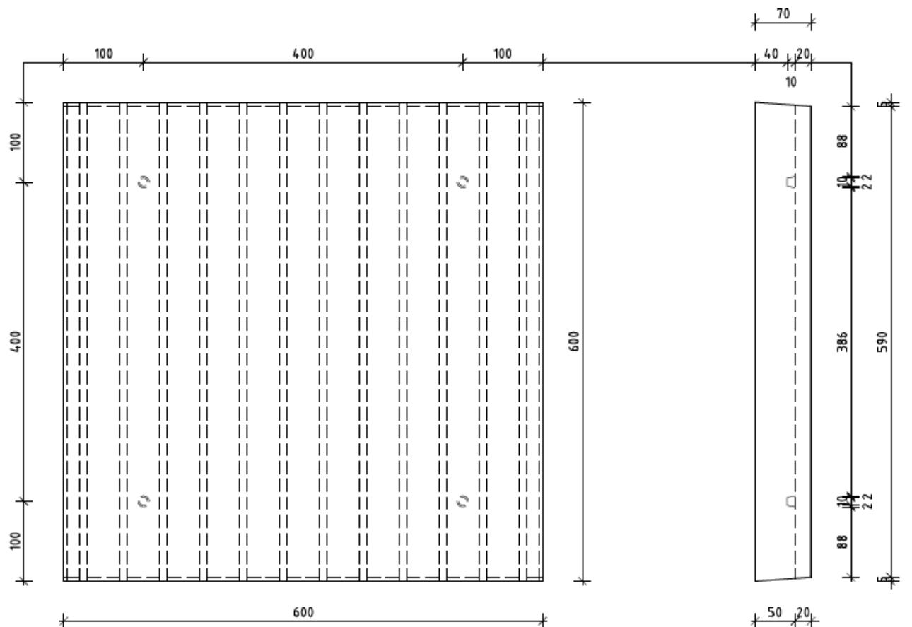
ZIJEAANZICHT
