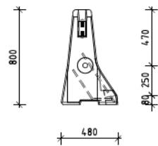
ZIJAANZICHT SCHAAL 1:25
