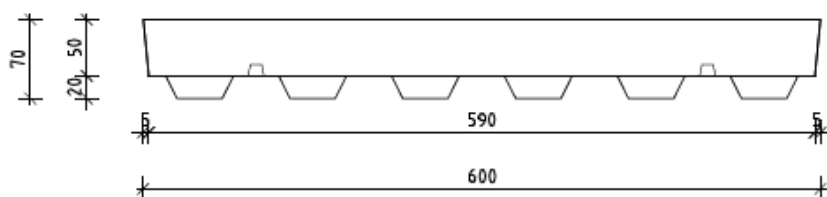
VOORAANZICHT
