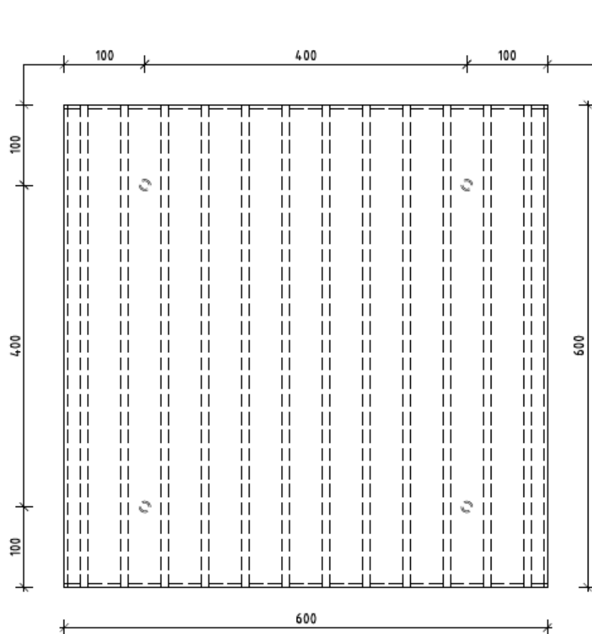
STORTAANZICHT
