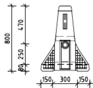
ZIJAAANZICHT SCHAAL 1:25
