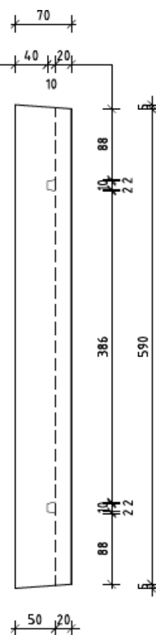
ZIJAANZICHT
