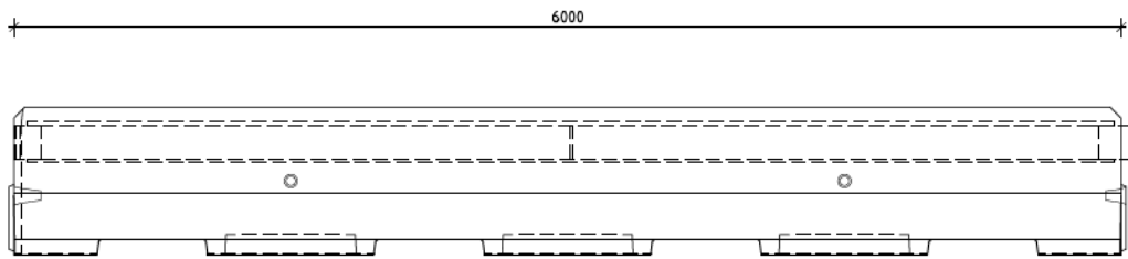
VOORAANZICHT SCHAAL 1:25
